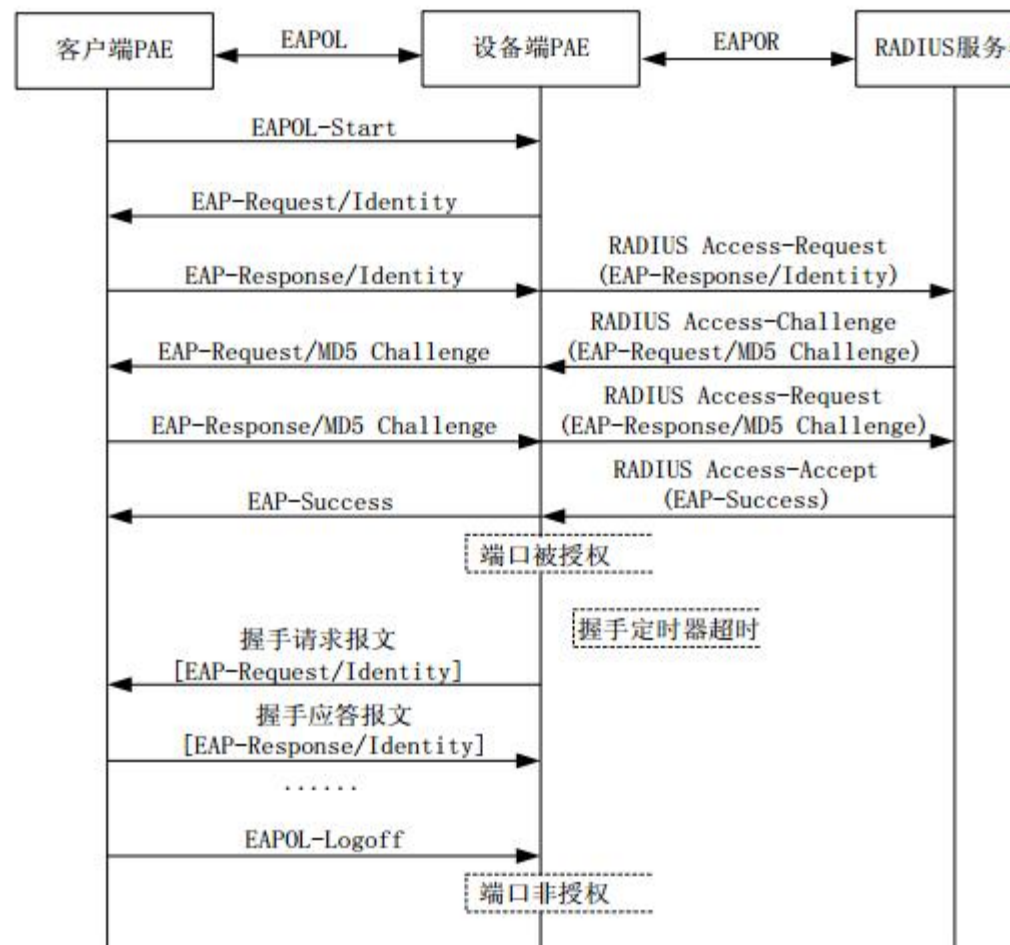
IEEE 802.1X 认证系统的 EAP 方式业务流程
